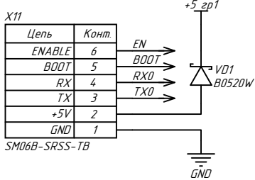
Программатор
