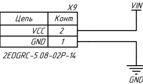
Вход питания
