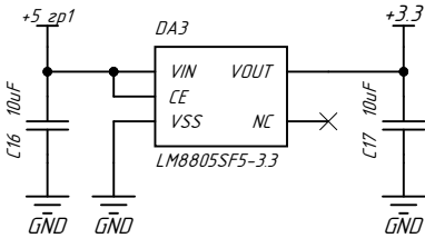
Питание MCU
